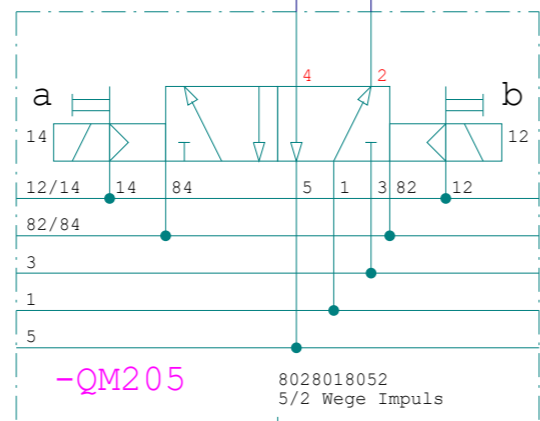
Druckumschaltung Kopfverschiebung
