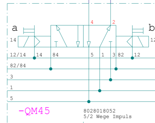
Druckumschaltung Spanner Stab BD
