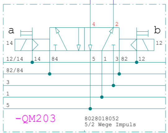
Riegel Kopfverschiebung
