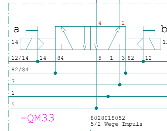
Werkzeuganhebung
