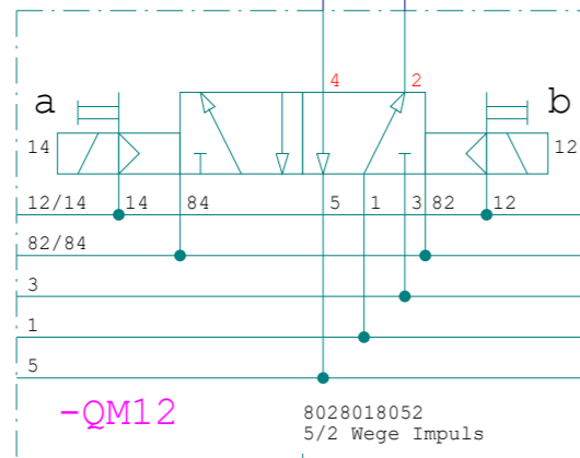
Abtransport Ausheber
