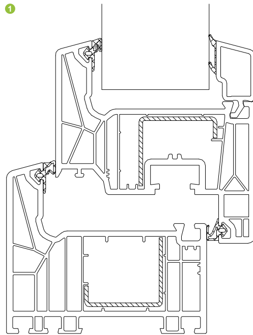
Schüco LivIng 82 AS mit Stahl 20271500 und 20271500 Prüfbericht 15-002325-PR 26 Schüco LivIng 82 AS with steel 20271500 and 20271500 Test report 15-002325-PR26
