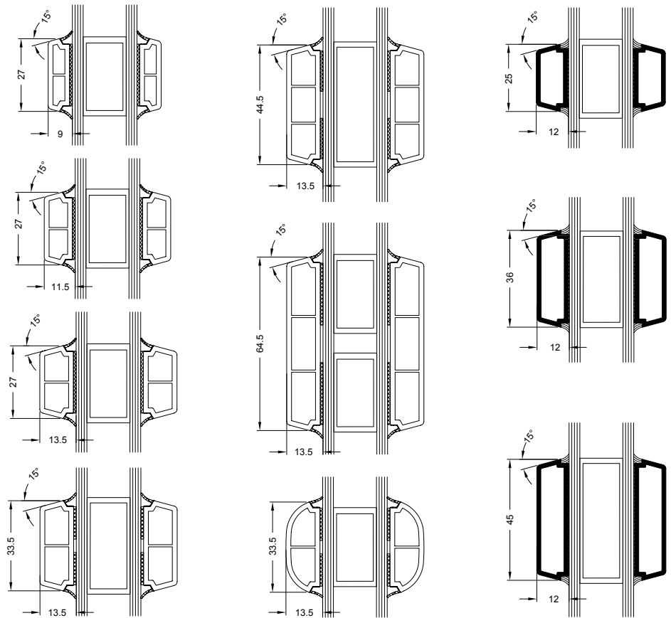
Maßstab 1:2 Scale 1:2
