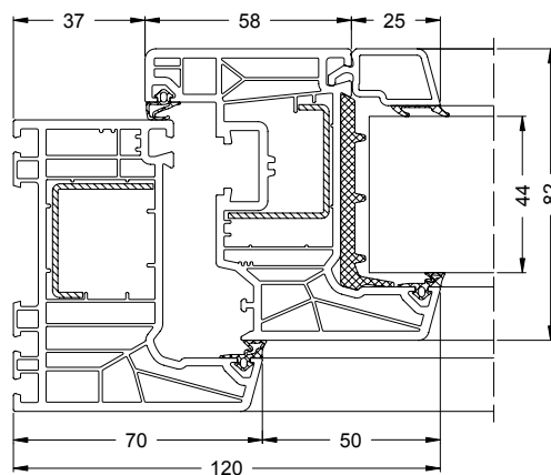
Schnitt Schüco LivIng 82 AS mit Dämmfalzeinleger 67 LivIng Section detail for Schüco LivIng 82 AS with LivIng insulating rebate insert 67
