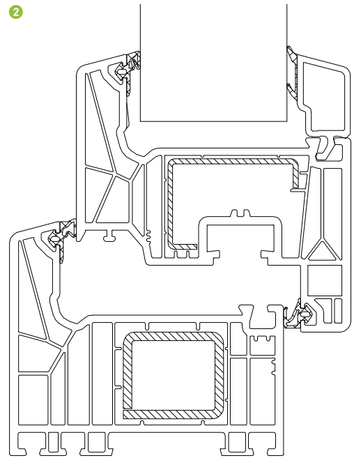
Schüco LivIng 82 AS mit Stahl 20271900 und 20272500 Siehe Prüfbericht System U-Wert Schüco LivIng 82 AS with steel 20271900 and 20272500 See U value test report for system
