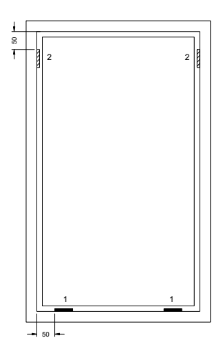
Festverglasung Fixed glazing
